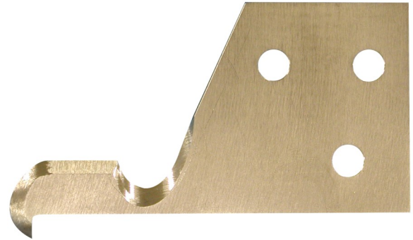
ブレードカッター(50×30×1mm)
